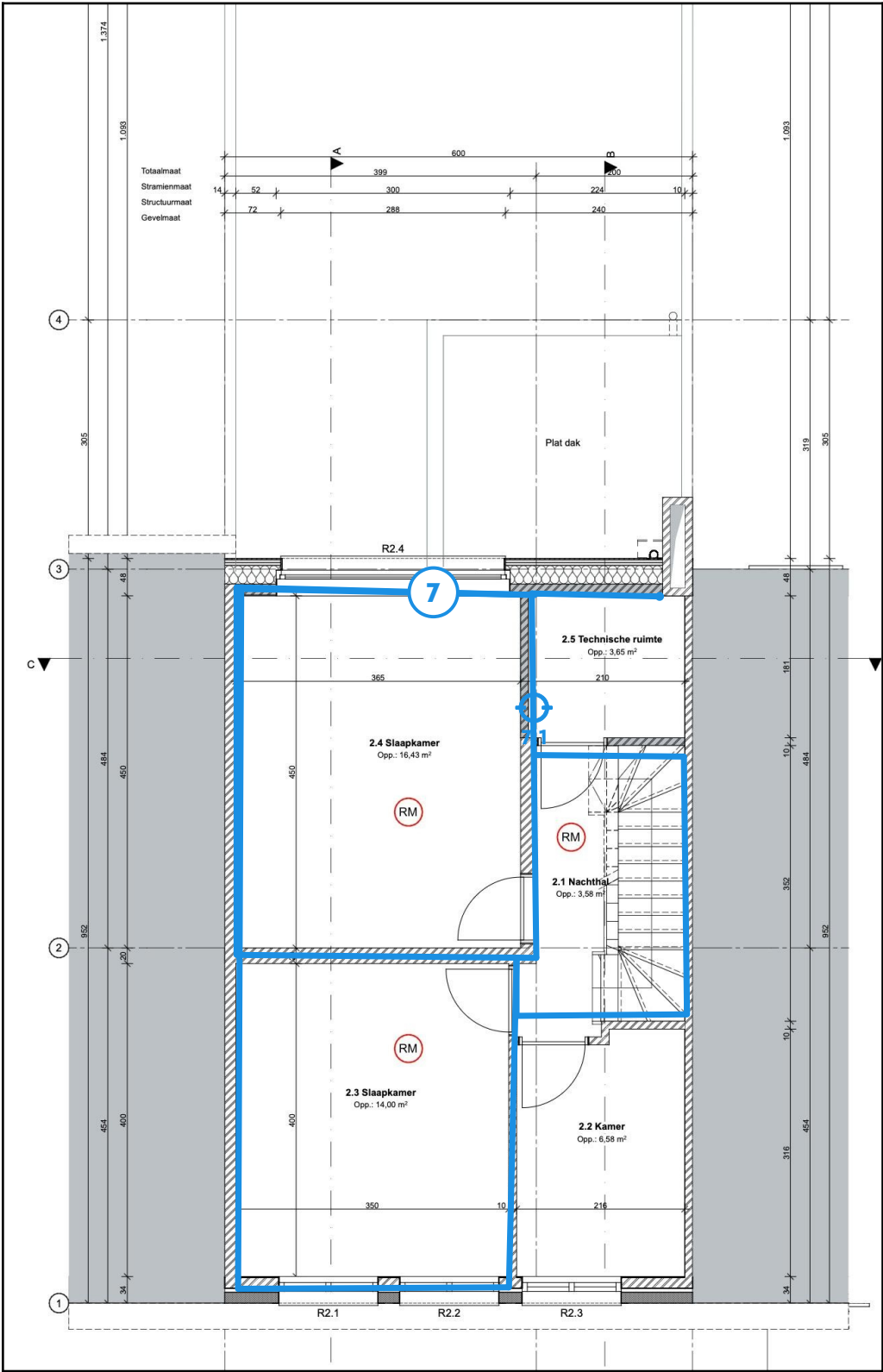
Legende van plan 1.10: Plan woning +2
