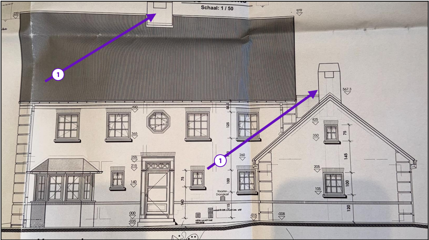
Legende van plan 1.8: Vooraanzicht woning
